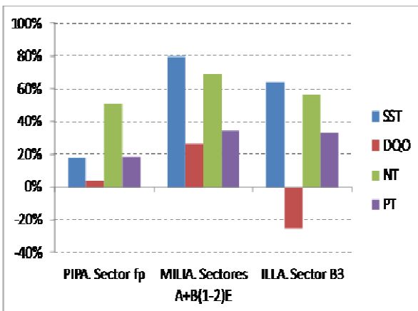
Fig. 1.- Porcentajes de reducción de concentraciones en los humedales artificiales.
